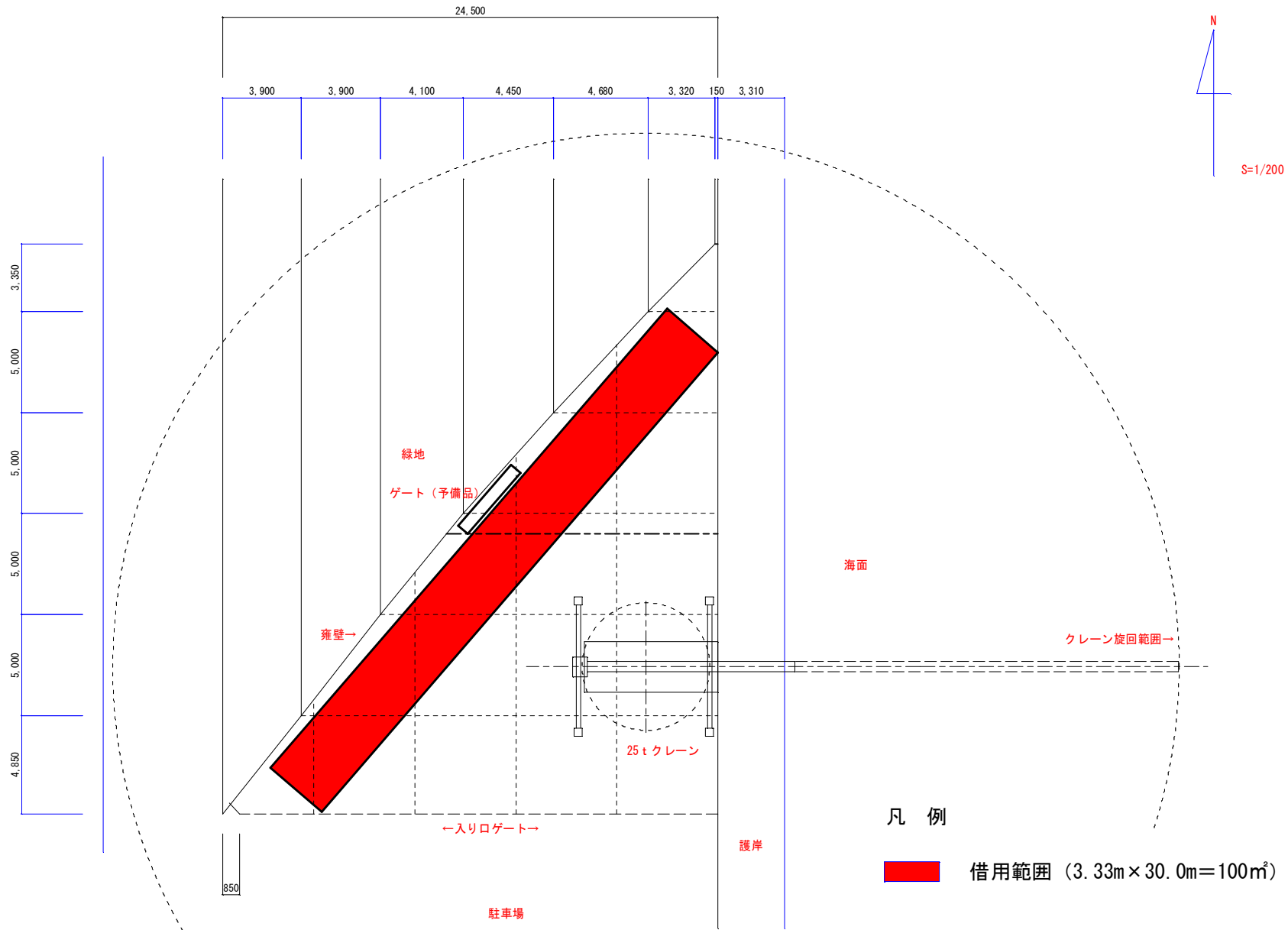
脇田漁港フィッシャリーナ整備用地平面図 財産の位置見取図
